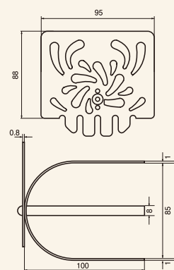
花柄ストレーナ
