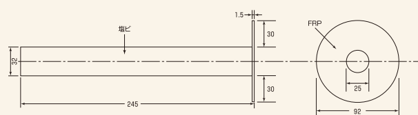
ダモオーバーフロー管TO-25
