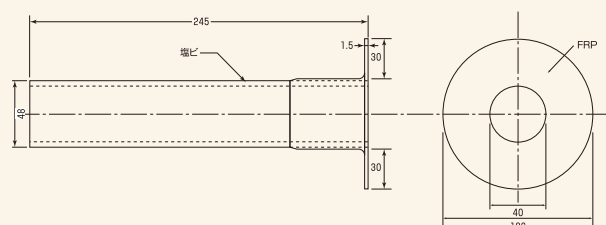
ダモオーバーフロー管TO-40
